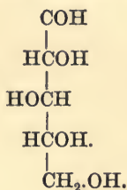
l. xylose.
